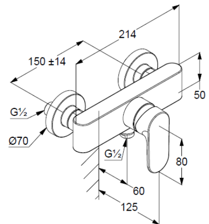
Maßzeichnung/ Dimensional drawing
